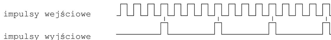
Rys. 7-2. Schemat operacji dzielenia częstotliwości przez 4
