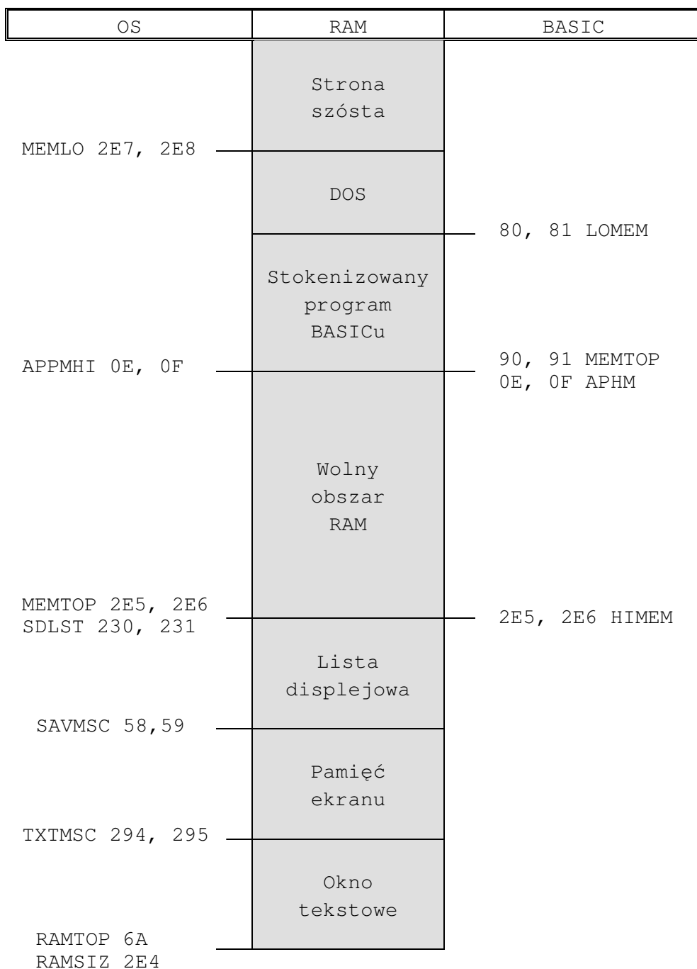
Rys. 8-2. Rejestry wskaźnikowe OS i BASICu.
