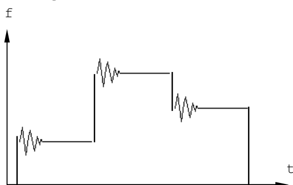
Rys. 7-13. Sekwencja zmian częstotliwości w brzmieniu fortepianu
